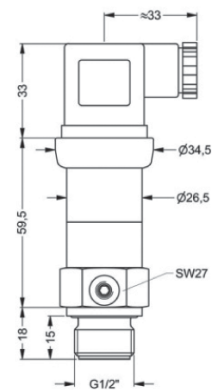
G1/2" flush DIN 3852
