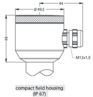
DIN 43650 A 1/2" NPTF conduit fitting
