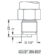
G1/2" EN 837
